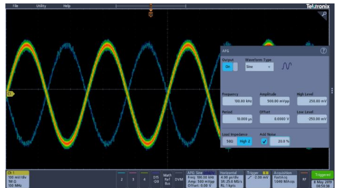
灵活设置 AFG 输出。在这个测试用例中，正弦波形中增加了 20% 的噪声。
