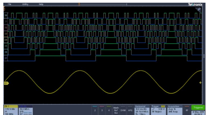
3 系列 MDO 及 3-MSO 选项通过同时探测模数转换器的两面，同时查看模拟信号和数字信号。
